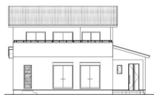
南側立面図
