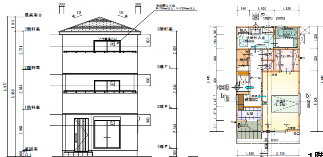
南側立面図
