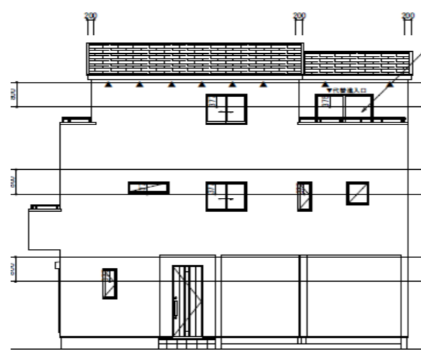
南側立面図
