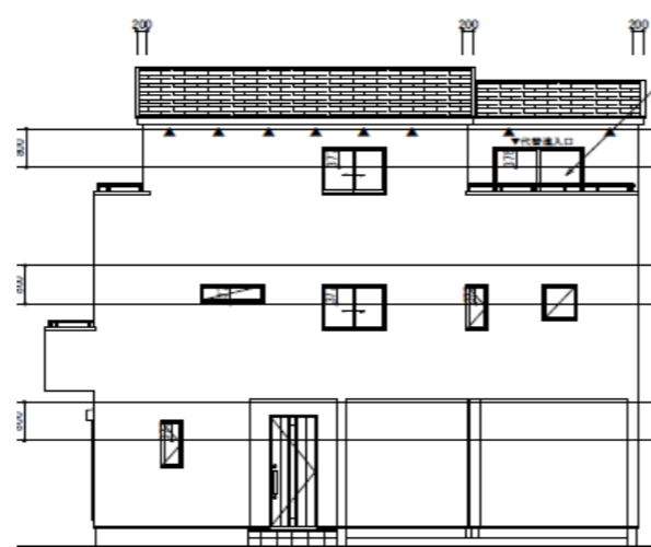
南側立面図
