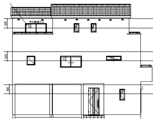
南側立面図
