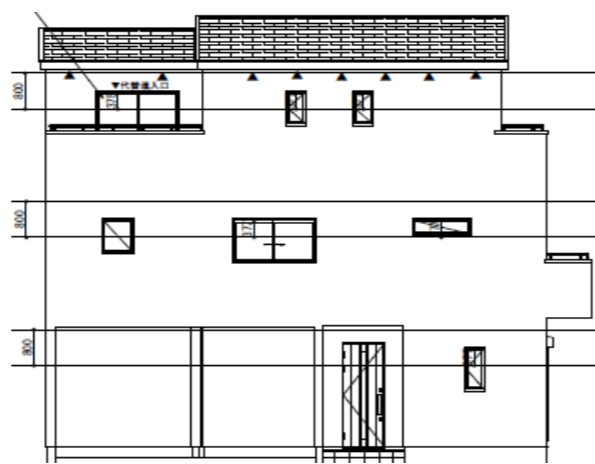
南側立面図
