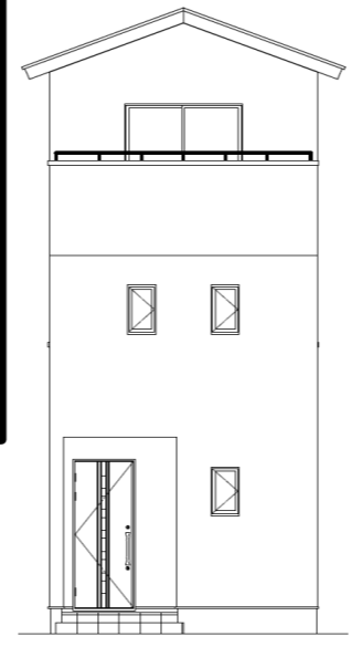
北側立面図
