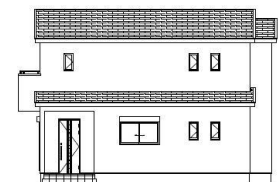
東側立面図
