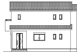
東側立面図
