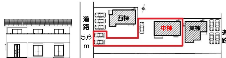
南側立面図
