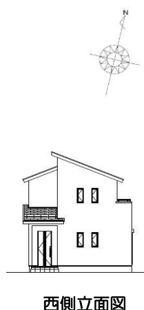
西側立面図
