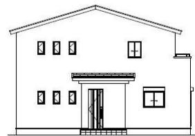
西側立面図
