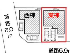
＜配置図＞
