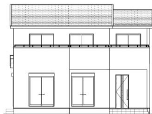
南側立面図
