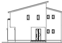
東側立面図
