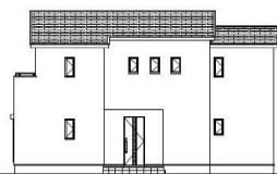
東側立面図
