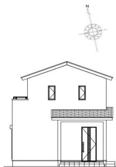
東側立面図
