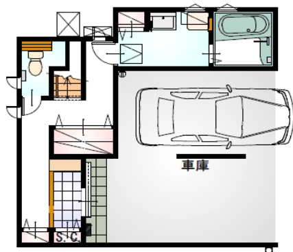
1階 車庫(27.32㎡)
