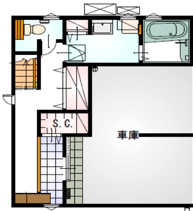
1階 車庫(22.36㎡)
