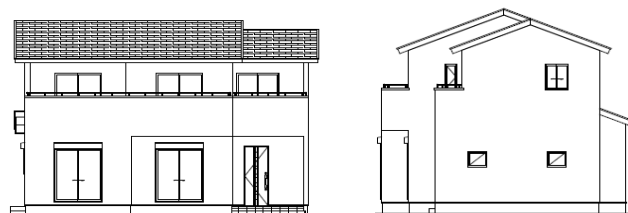
《南側立面図》
