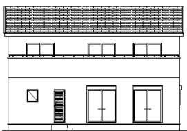
《南側立面図》
