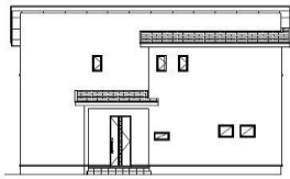
《北側立面図》
