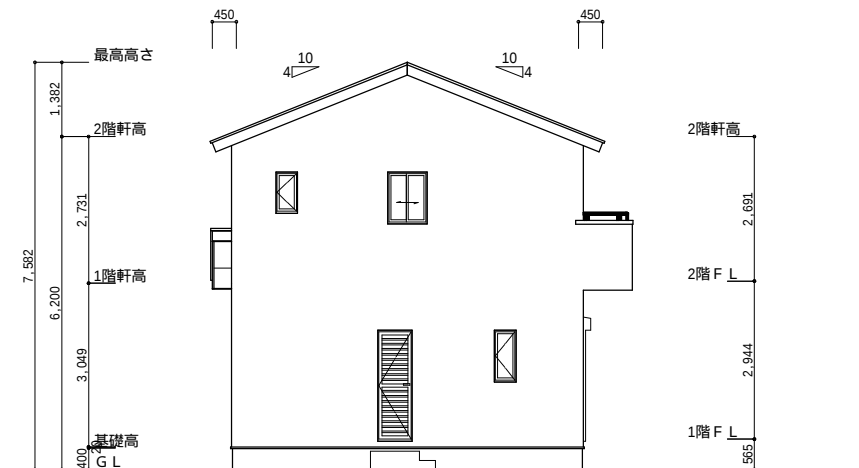
西側 立面図 S:1/100
