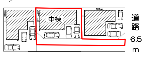
《3棟配置図》
