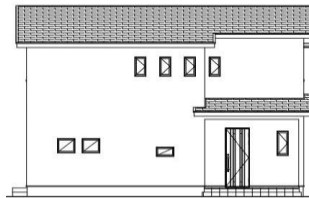
北側立面図
