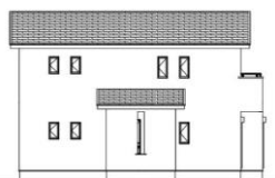
西側立面図
