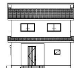
北側立面図
