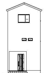
北側立面図
