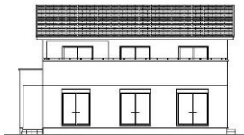
《南側立面図》
