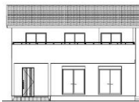
南側立面図
