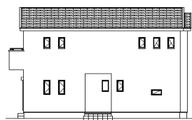
《東側立面図》
