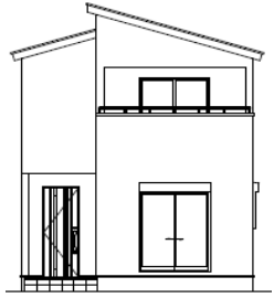
《南側立面図》
