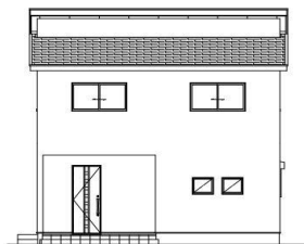
北側立面図
