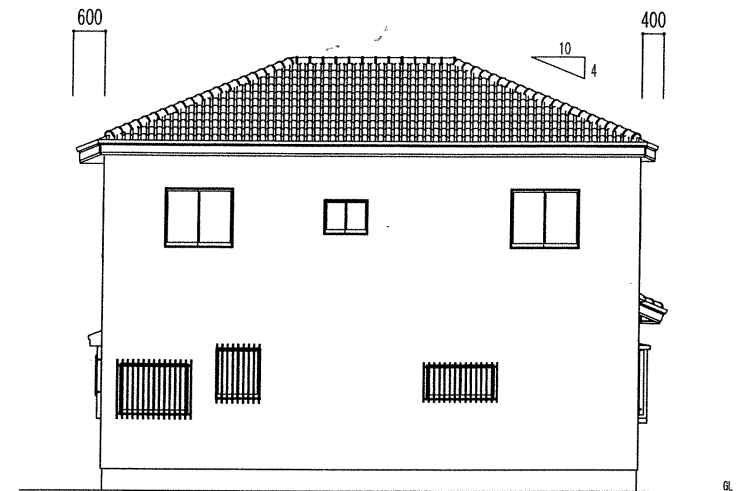
東側立面図 1/100
