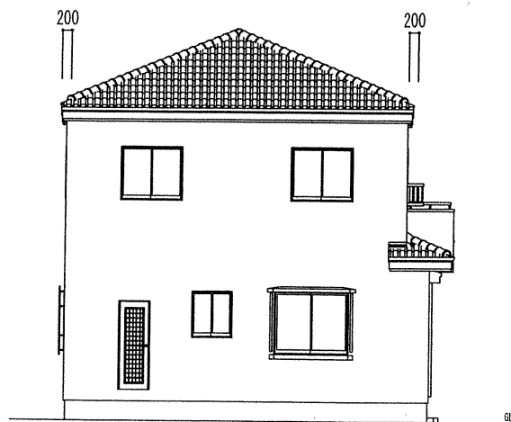
北側立面図 1/100
