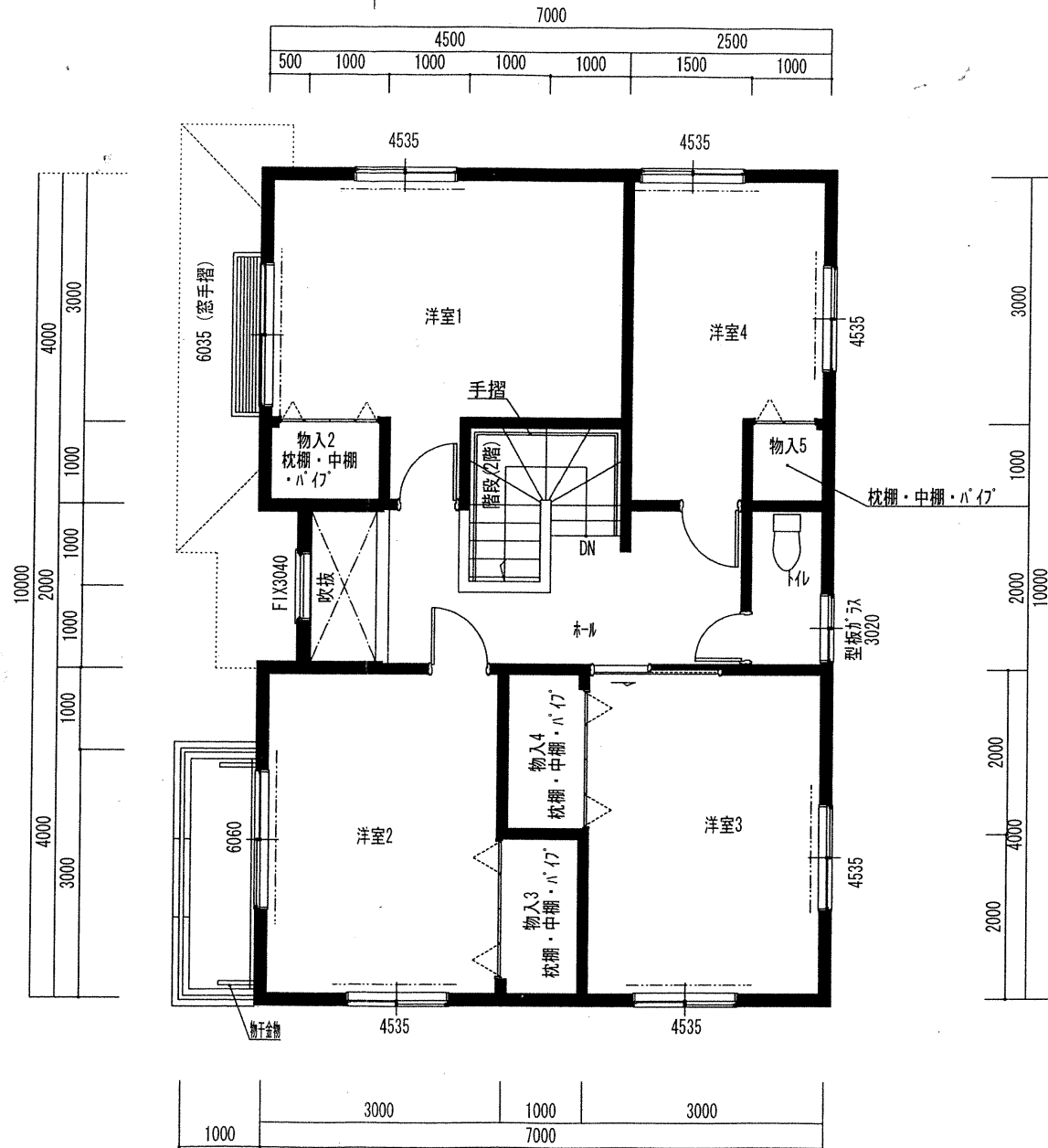
2階平面図 1/60
