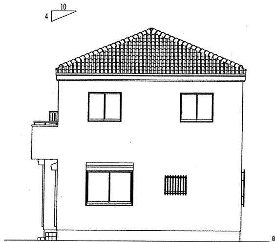
南側立面図 1/100
