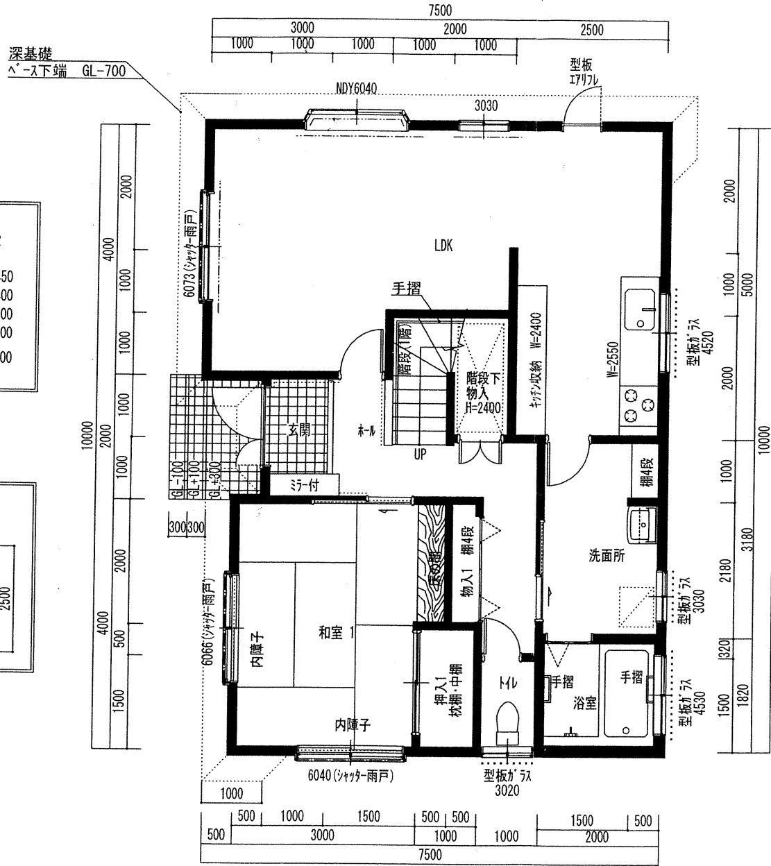
1階平面図 1/60
