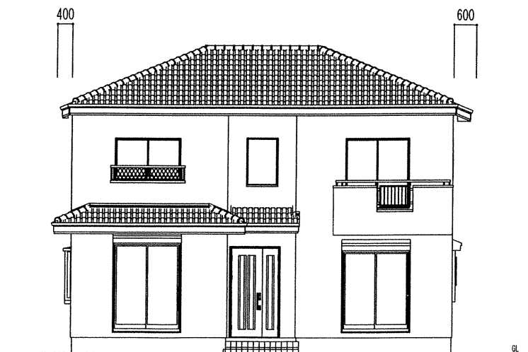
西側立面図 1/100
