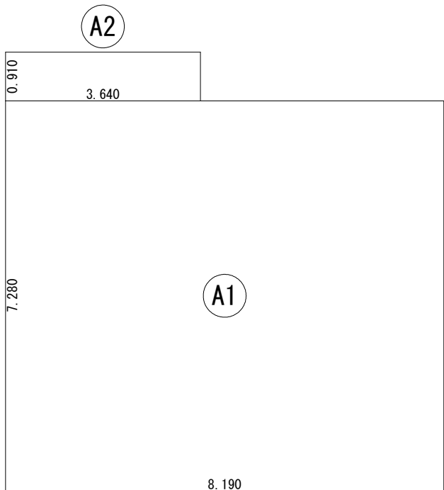
建築面積求積図 S:1/100
