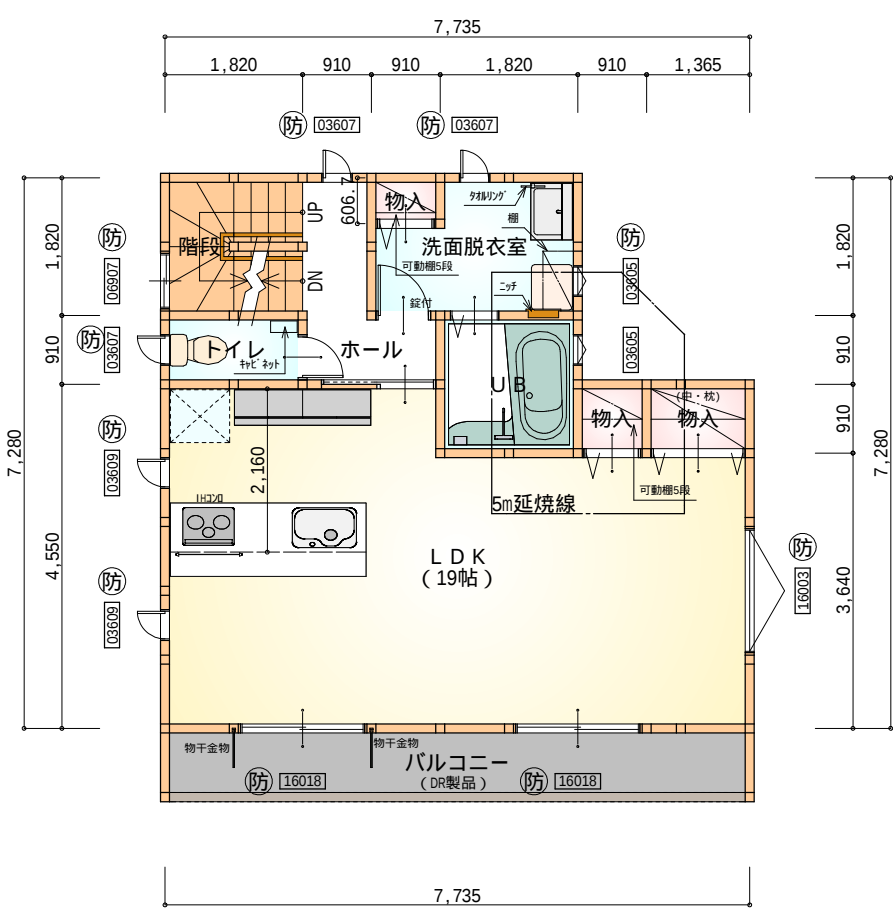
令第120条における居室から 階段までの歩行距離50m以内
