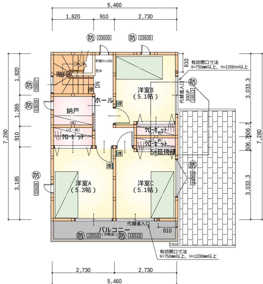
令第120条における居室から 階段までの歩行距離50m以内
