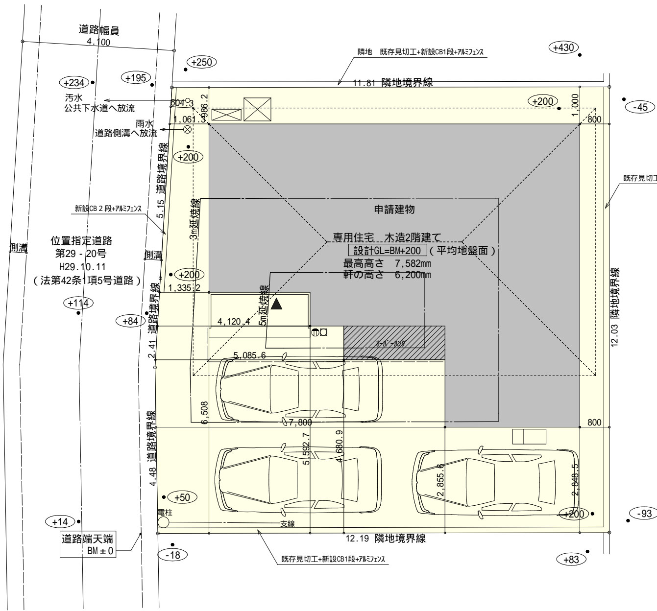
配置図 S:1/100
