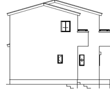
《西側立面図》
