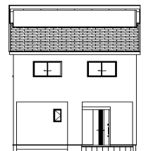
《北側立面図》
