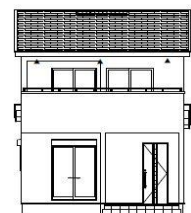
南側立面図
