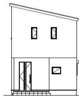
北側立面図
