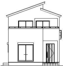
南側立面図
