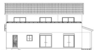
南側立面図
