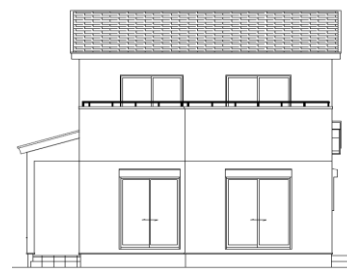
《南側立面図》
