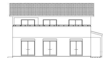
《南側立面図》
