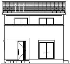
南側立面図
