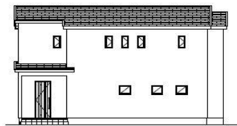
《北側立面図》
