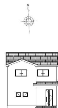
≪北側立面図≫
