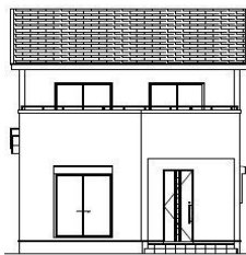
《東側立面図》
