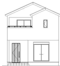
《南側立面図》
